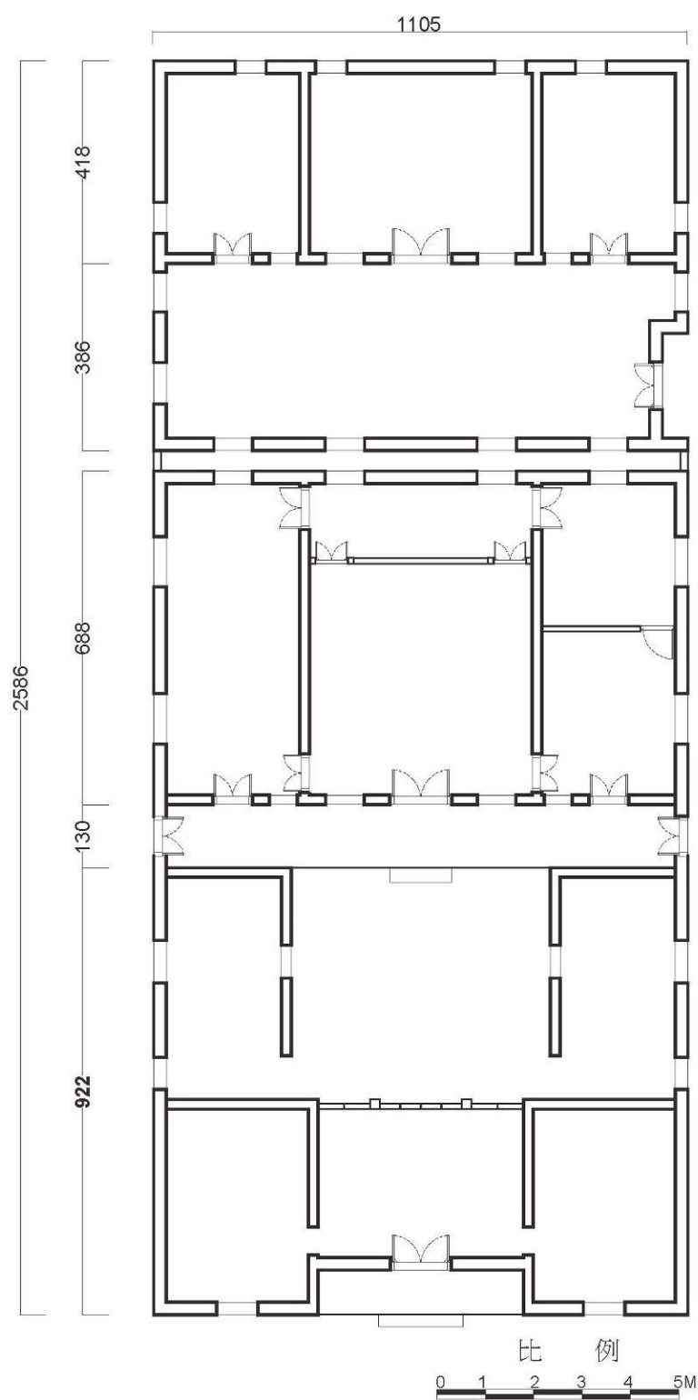
湖下楊允泡及楊盤讀古厝—建築平面圖
