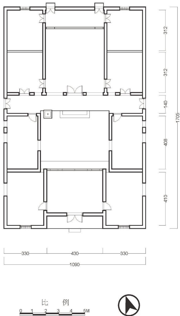
圖四、後浦東門境洪氏古厝－建築平面圖
