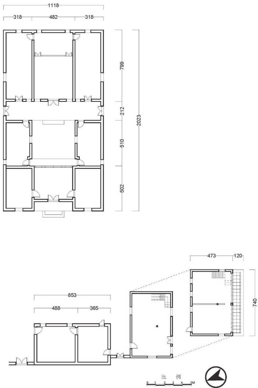
圖四、浦邊周文獻古曆—建築平面圖
