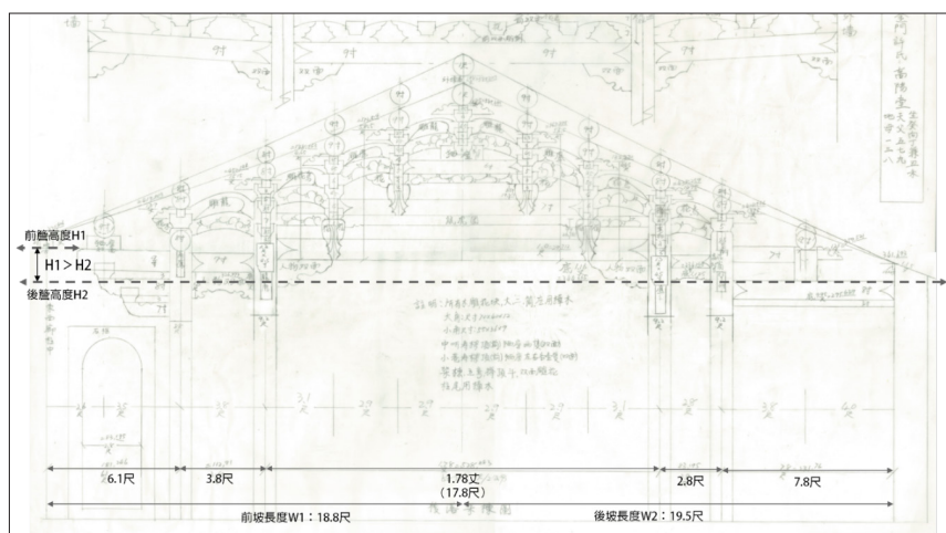
圖72 陰陽坡、前高後低（許氏高陽堂）
