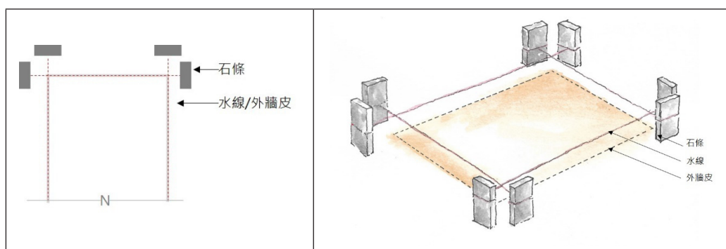
【圖19】 「石條」放樣方式
