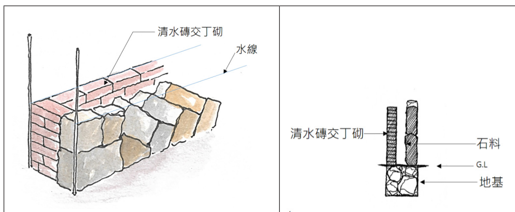
【圖30】砌至約二勻的高度後，暫停石砌，先作內牆磚砌
