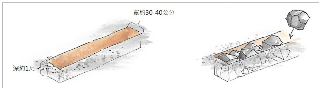
【圖21】自「外牆皮」向內約30-40公分，向下挖深度約1尺，若不是不良土必須挖至硬地
