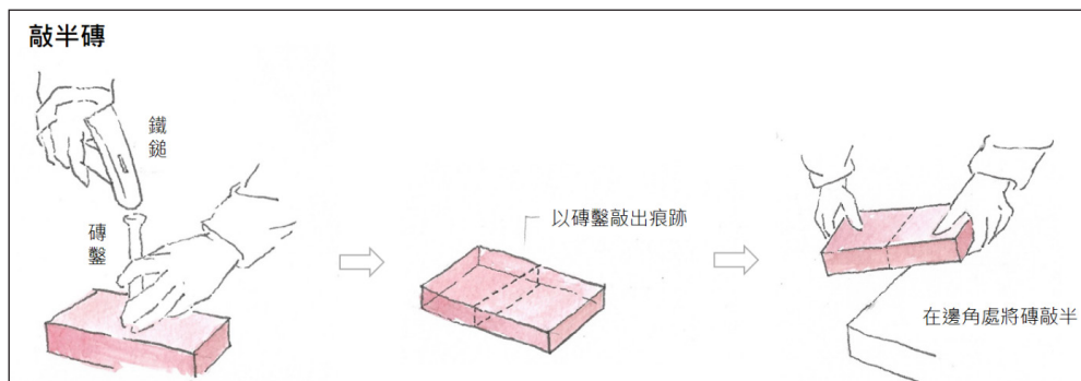
【圖43】敲半磚
