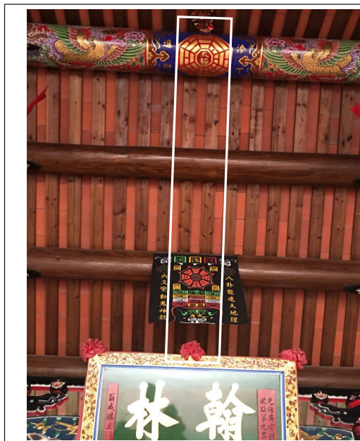
圖89 分金線兩側的桷木選用「目」 數量較多、左右對稱的木料 (頂堡翁氏家廟)
