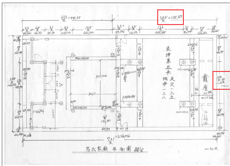
圖64 林兜呂氏宗祠地母尺寸
