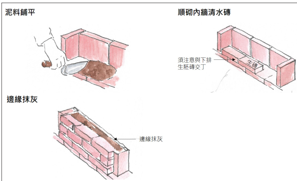
【圖45】順砌內牆清水磚
