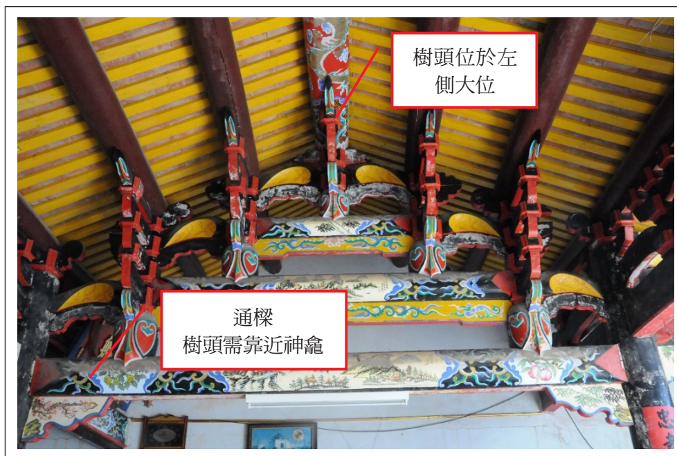
圖87 木料樹頭位置說明圖
