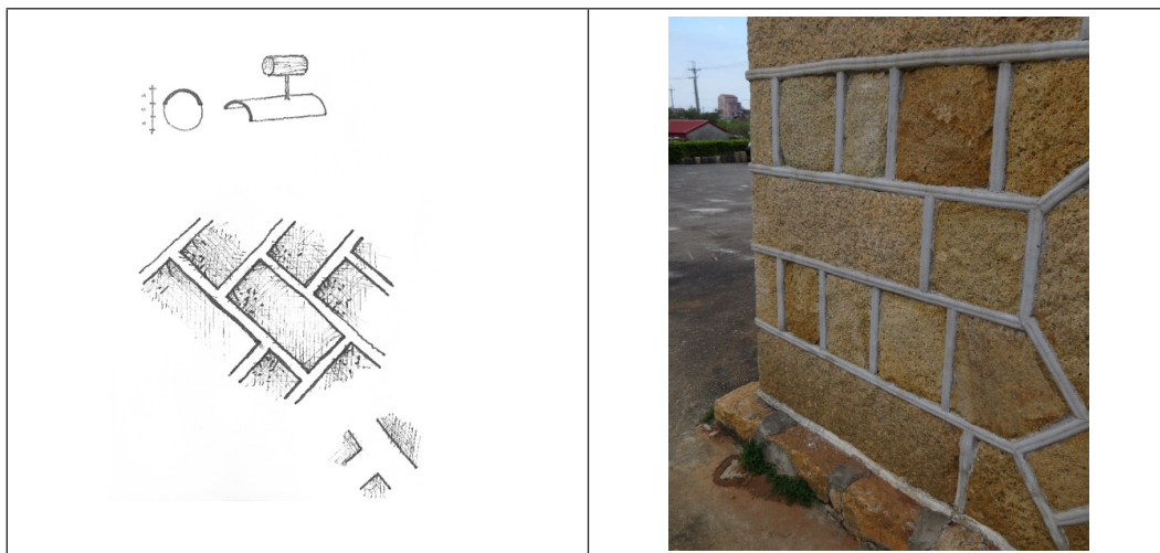
【圖35】於灰縫處填上蚵殼灰灰糲，以鐵管自製弧形灰匙拖拉灰糲塑形於石牆灰縫線上，所修飾灰縫交接處為「四角」，西司認為此種勾縫不甚好看
