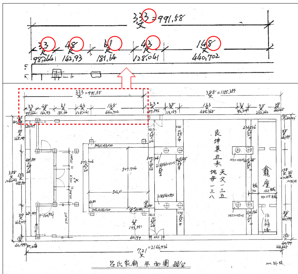
圖49 呂氏家廟前殿之地母寸白檢視
