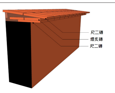
【圖62】出料作法（三勻）
