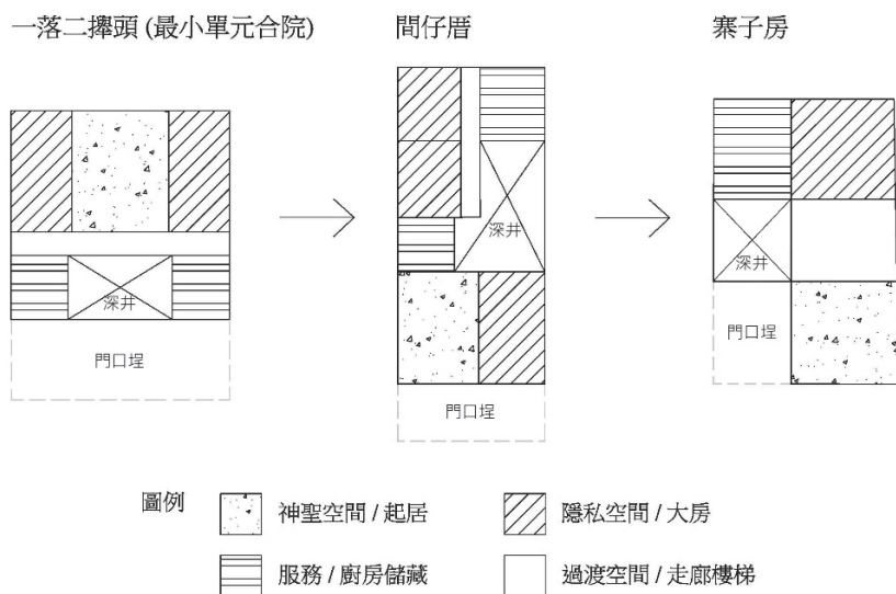
圖11 從小合院到間仔厝的平面演化
