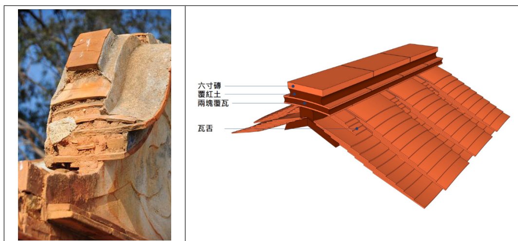
【圖69】馬路脊
