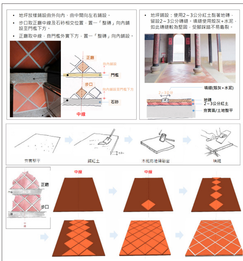
【圖78】地坪放樣及鋪設
