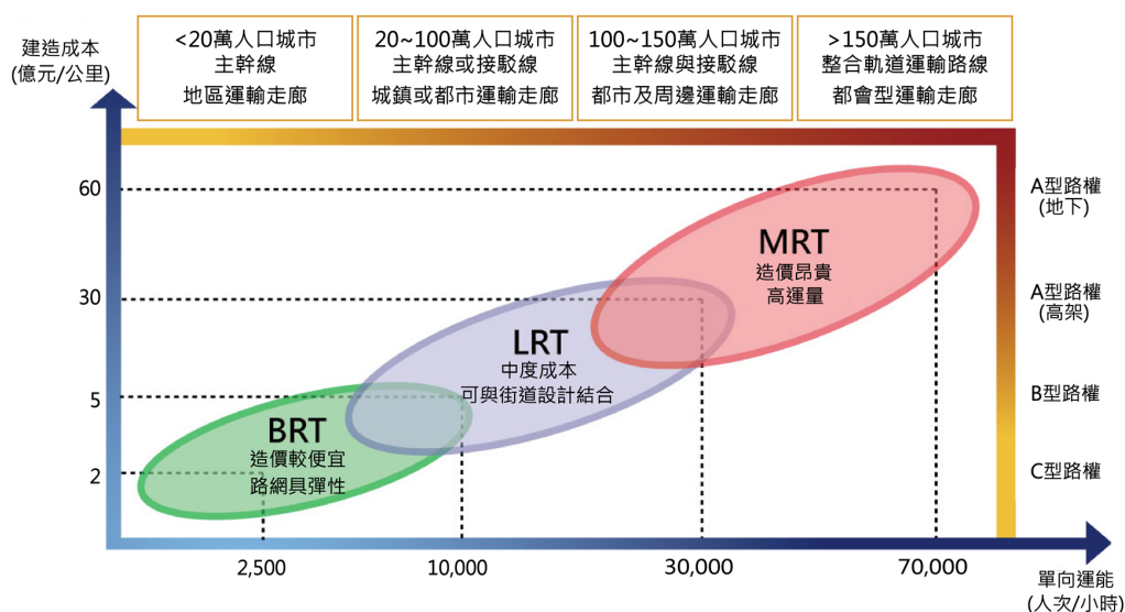
圖14 TOD基本運具特徵及適用都市規模之比較
