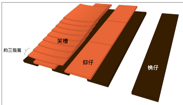
【圖74】莊西勢匠師笑槽瓦片取「三指寬」為間距
