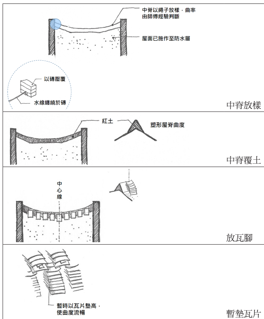
【圖65】屋頂中脊曲線作法
