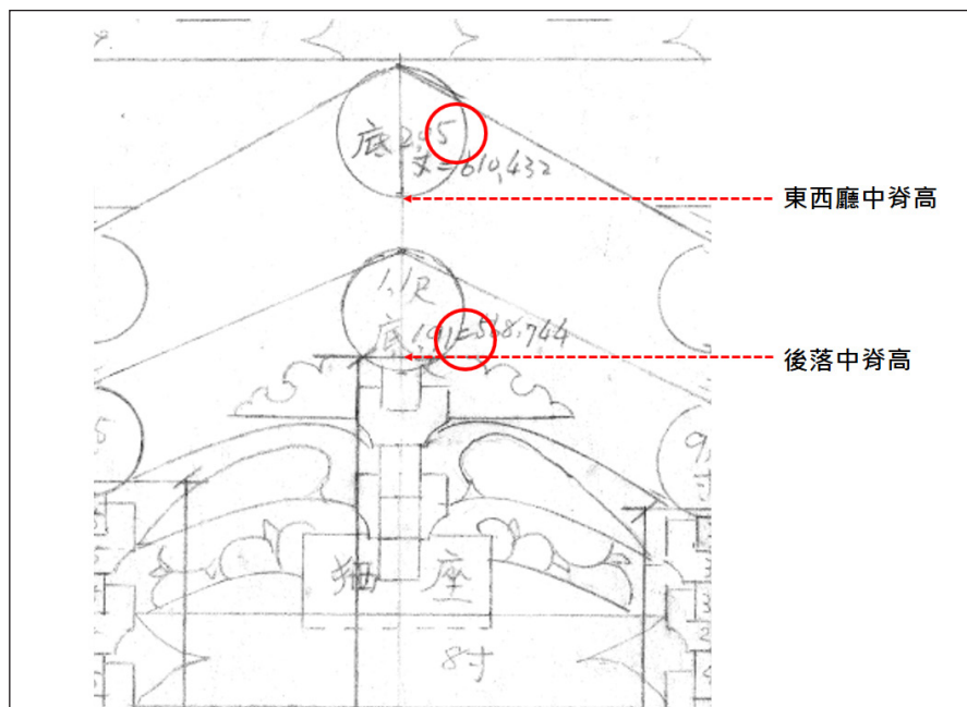
圖52 呂氏家廟後殿中脊及東西廳中脊天父寸白檢視
