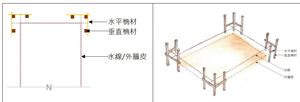
【圖20】 「三角架」放樣方式
