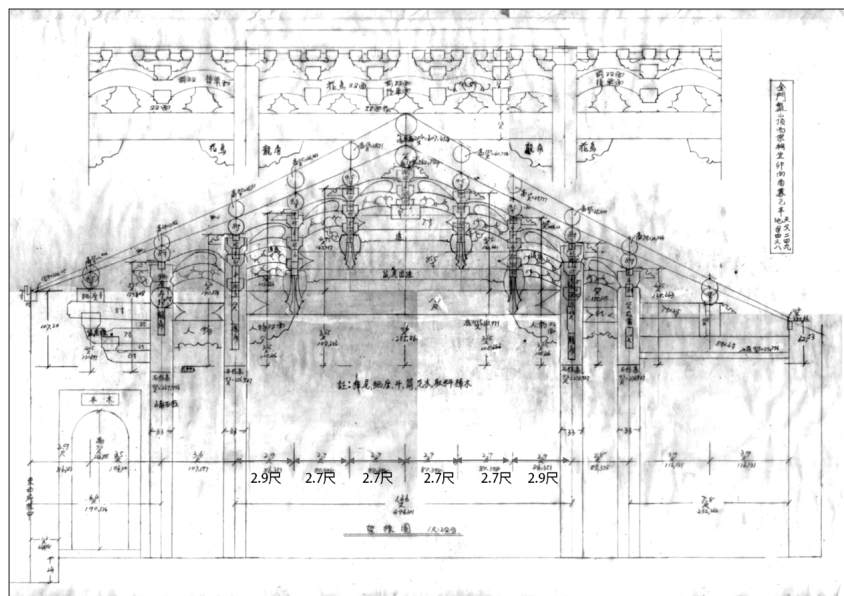
圖76 盤山頂西宗祠架內步步進（分縫尺寸）說明圖
