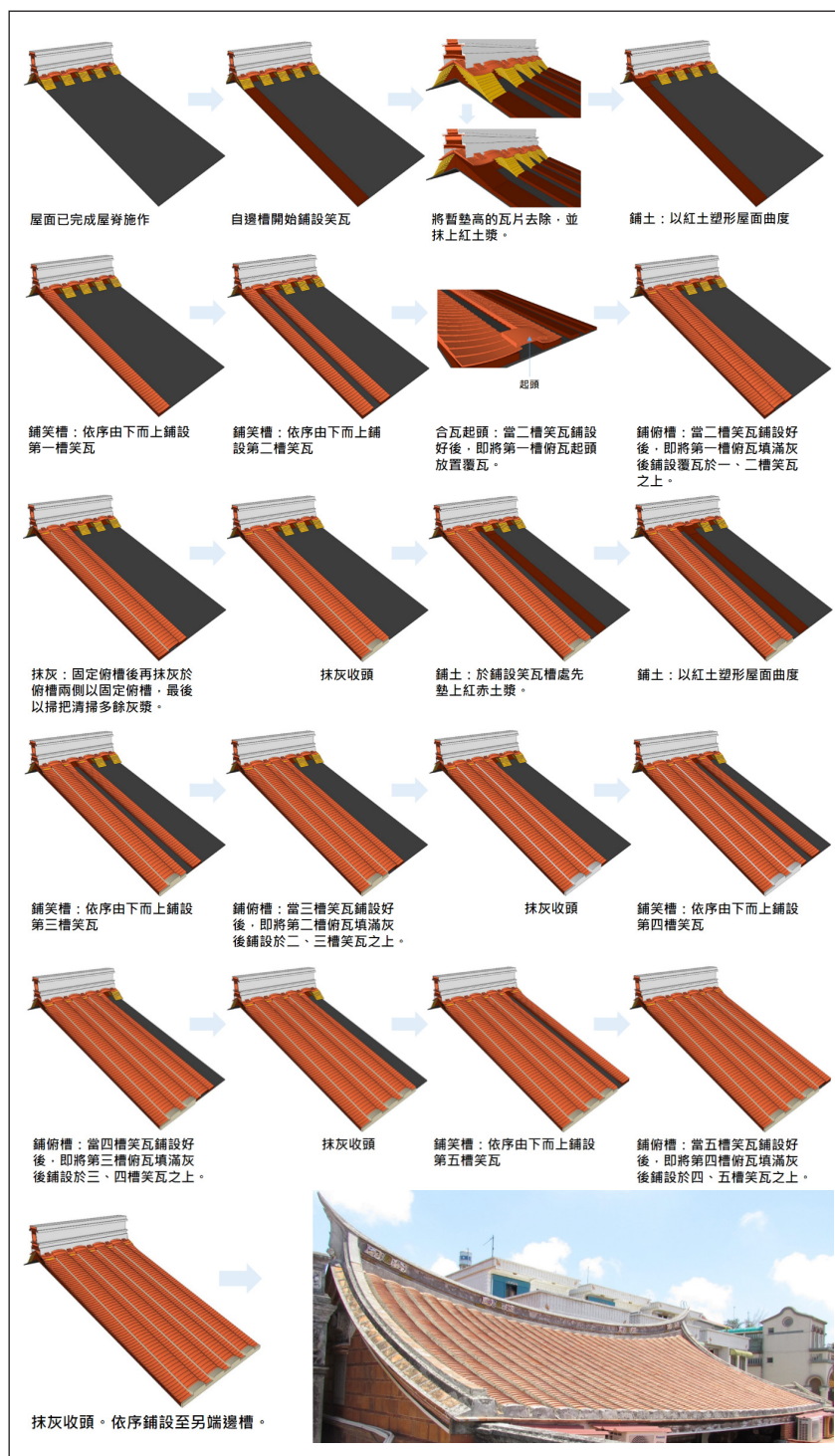
【圖75】鋪瓦步驟（1）
