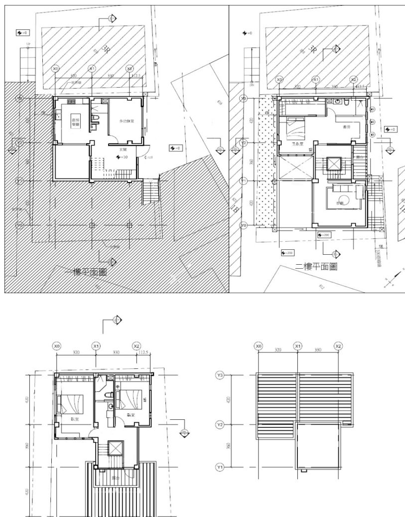
圖16 寨子房各層平面圖
