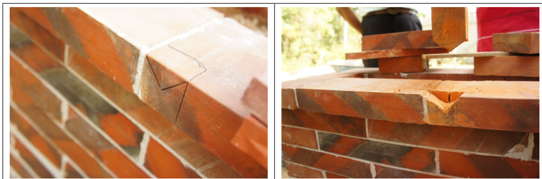
【圖53】收邊框料切割範圍
