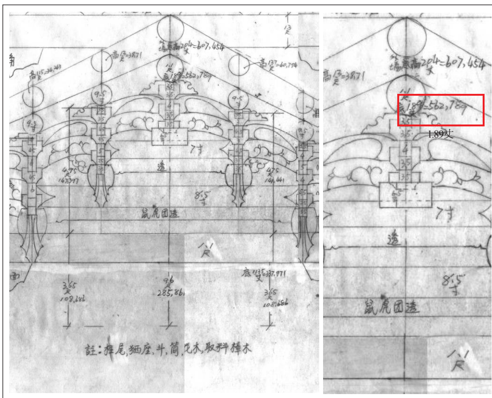
圖67 頂堡翁氏宗祠天父尺寸
