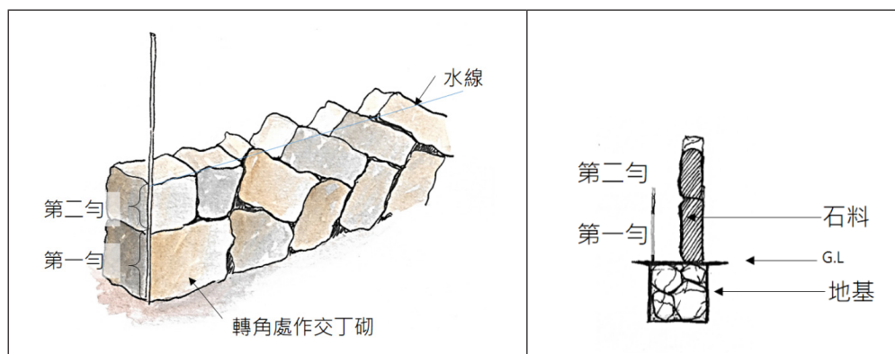
【圖29】依序砌作，轉角處先作交丁砌，再於中段作人字砌
