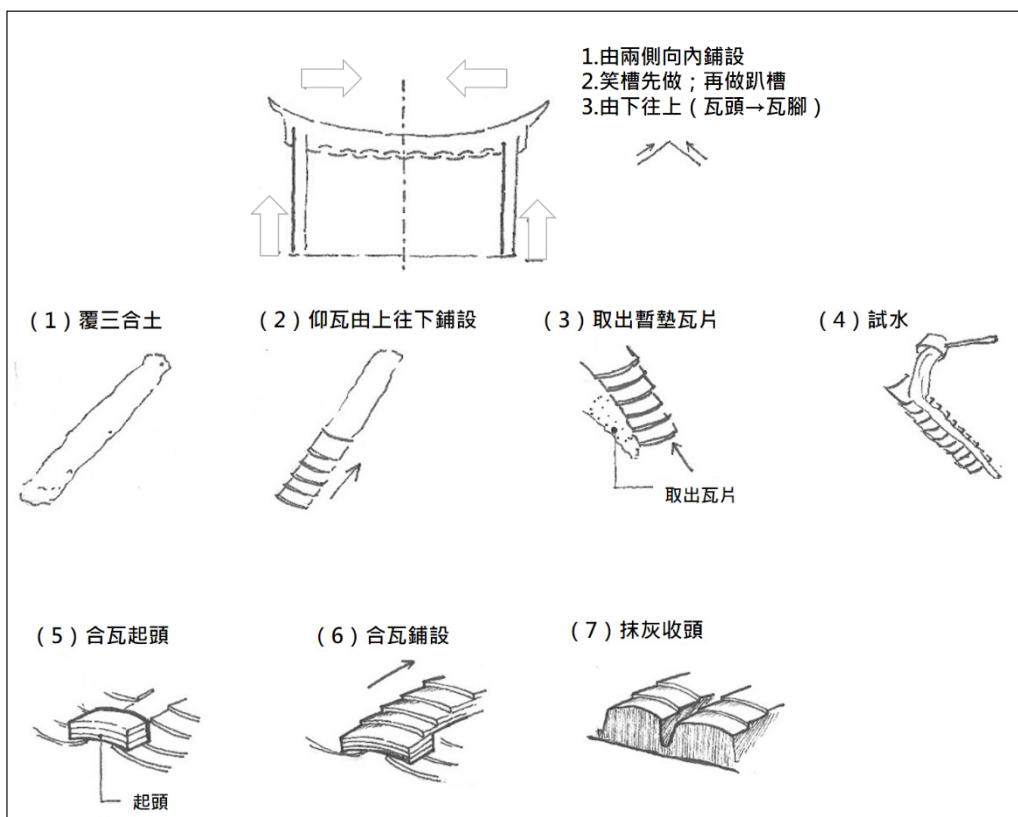
【圖76】鋪瓦步驟（2）
