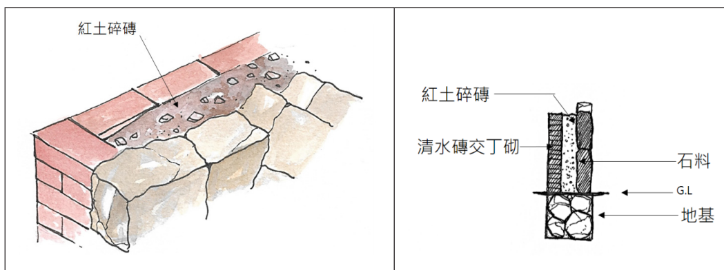
【圖31】磚石間填入紅土碎磚
