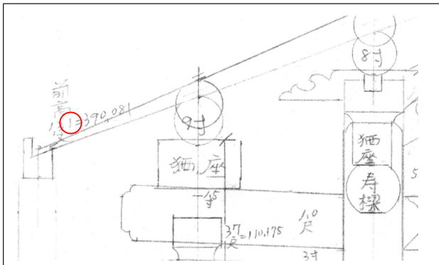
圖53 呂氏家廟後殿前簷口寸白檢視
