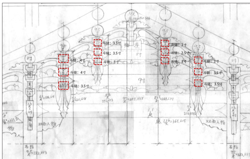
圖73 高陽堂架棟斗縫說明圖
