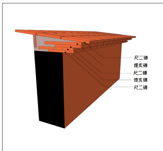
【圖63】出料作法（五勻）
