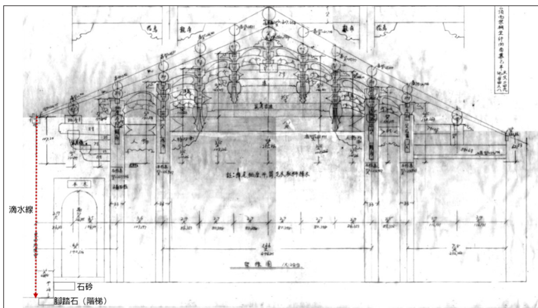
圖83 目屎流滴示意圖（翁氏宗祠）
