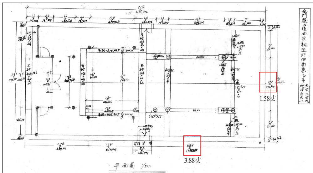
圖66 頂堡翁氏宗祠地母尺寸
