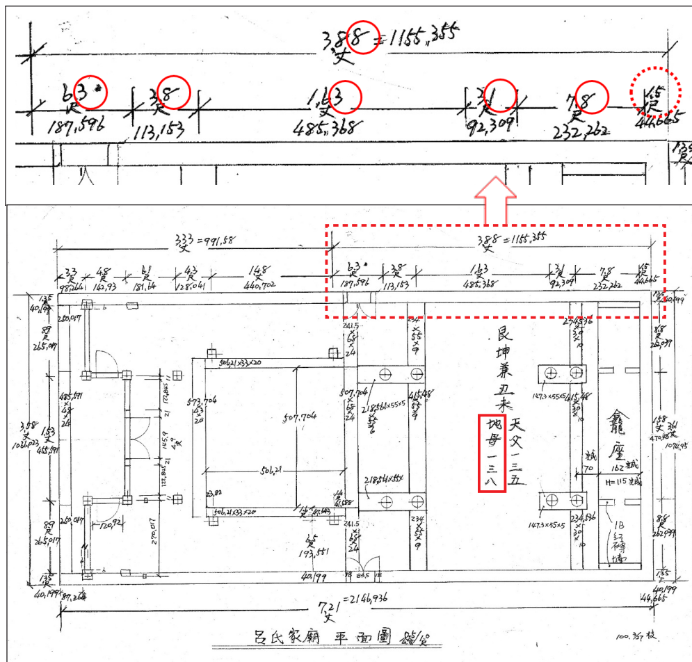
圖50 呂氏家廟後殿之地母寸白檢視
