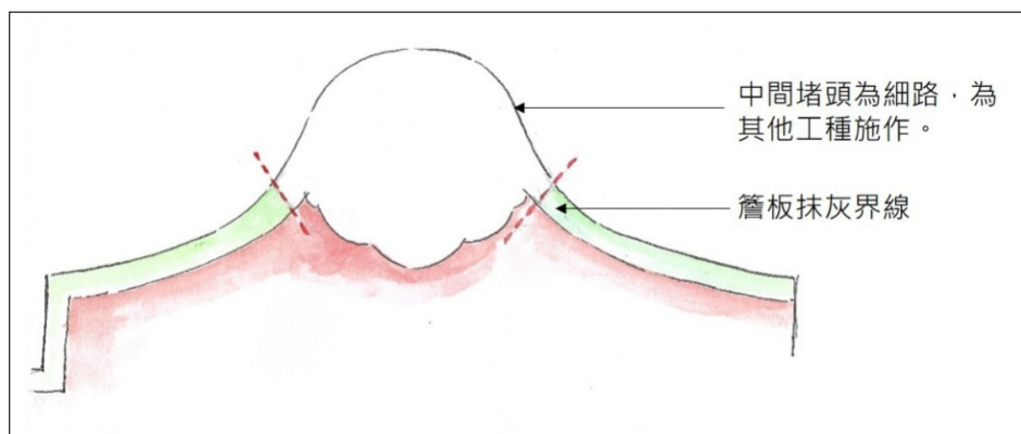
【圖58】圓規脊簷板灰作
