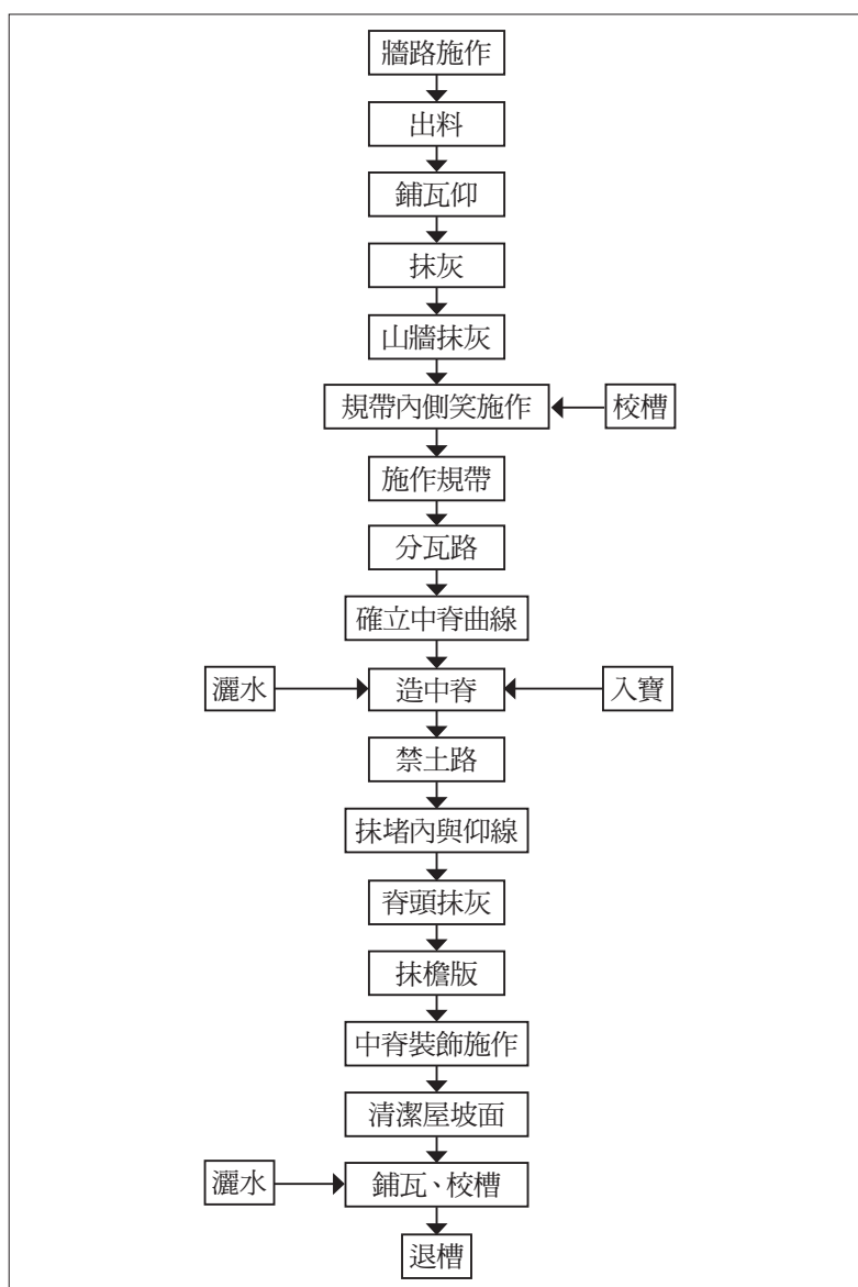
【圖60】莊西勢瓦作施作之流程
