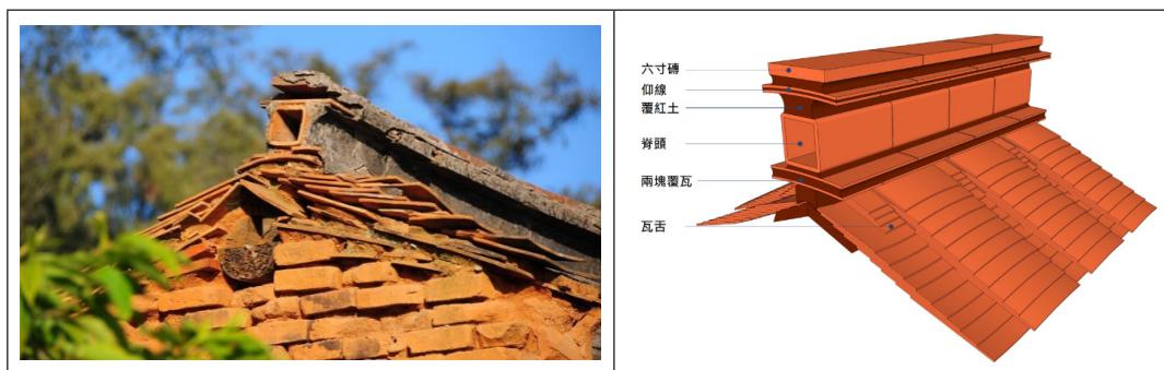
【圖67】小腹脊
