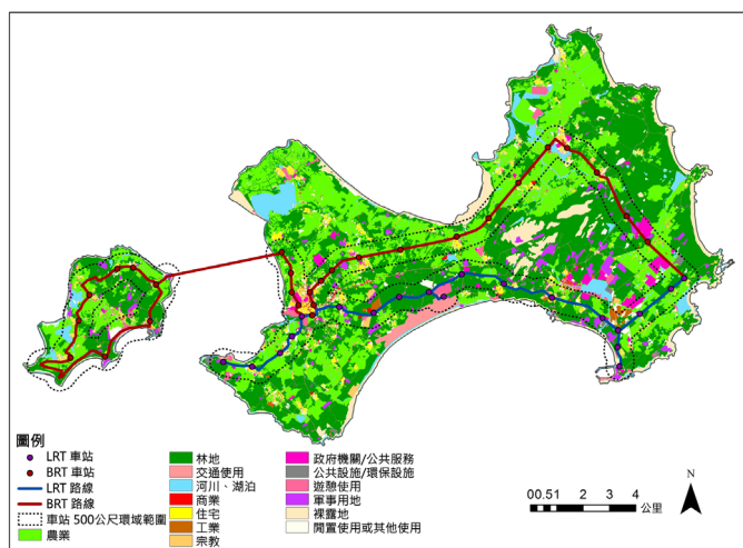
圖12 Green TOD方案A：輕軌和BRT結合的建議路線和站點
