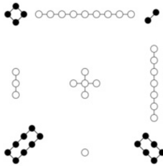
圖七 〈洛書〉九宮圖
