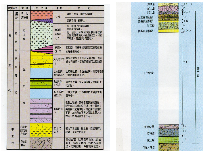
圖3 金門古河道地層結構圖 12
