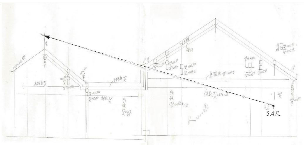
圖68 翁水千匠師圖繪符合見白（林兜呂氏宗祠）
