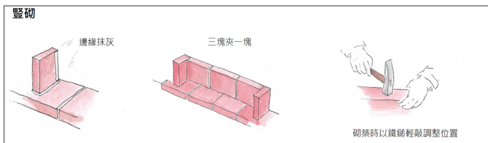
【圖44】豎砌
