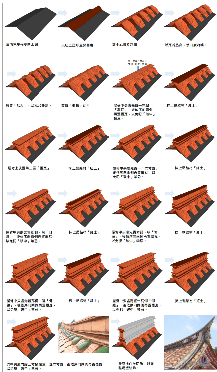
【圖70】脊樑施作步驟
