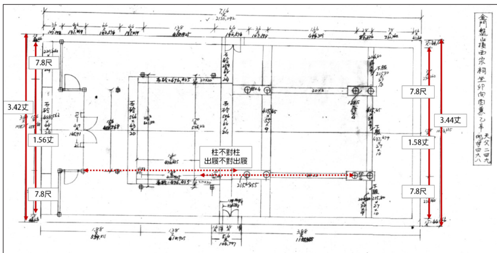
圖77 翁氏宗祠後包前、柱不對柱禁忌示意圖
