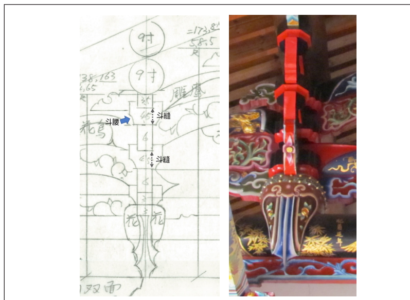
圖74 斗縫細部圖
