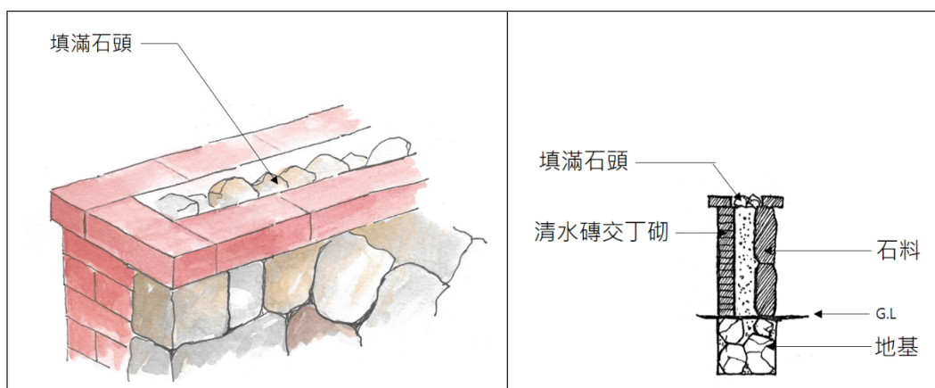
【圖33】以紅磚作石砌臺度，紅磚中間填入石頭
