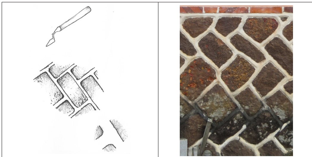
【圖34】以灰匙填滿蚵殼灰灰糲壓於石牆灰縫線上，所修飾灰縫交接處可見「彎角」特點，稱「手工」抹灰縫，為傳統作法（珠山大道公廟，莊西勢2013作品）
