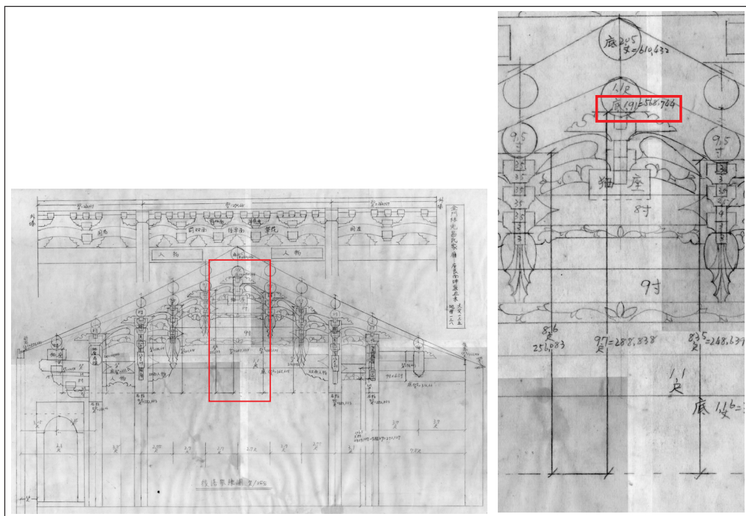
圖65 林兜呂氏宗祠天父尺寸
