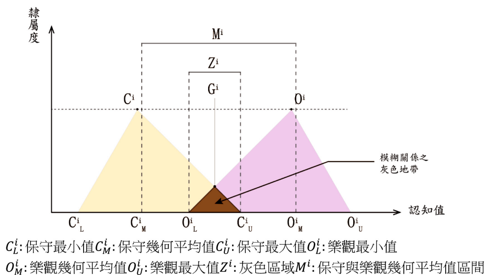
圖1 雙三角模糊樹示意圖
