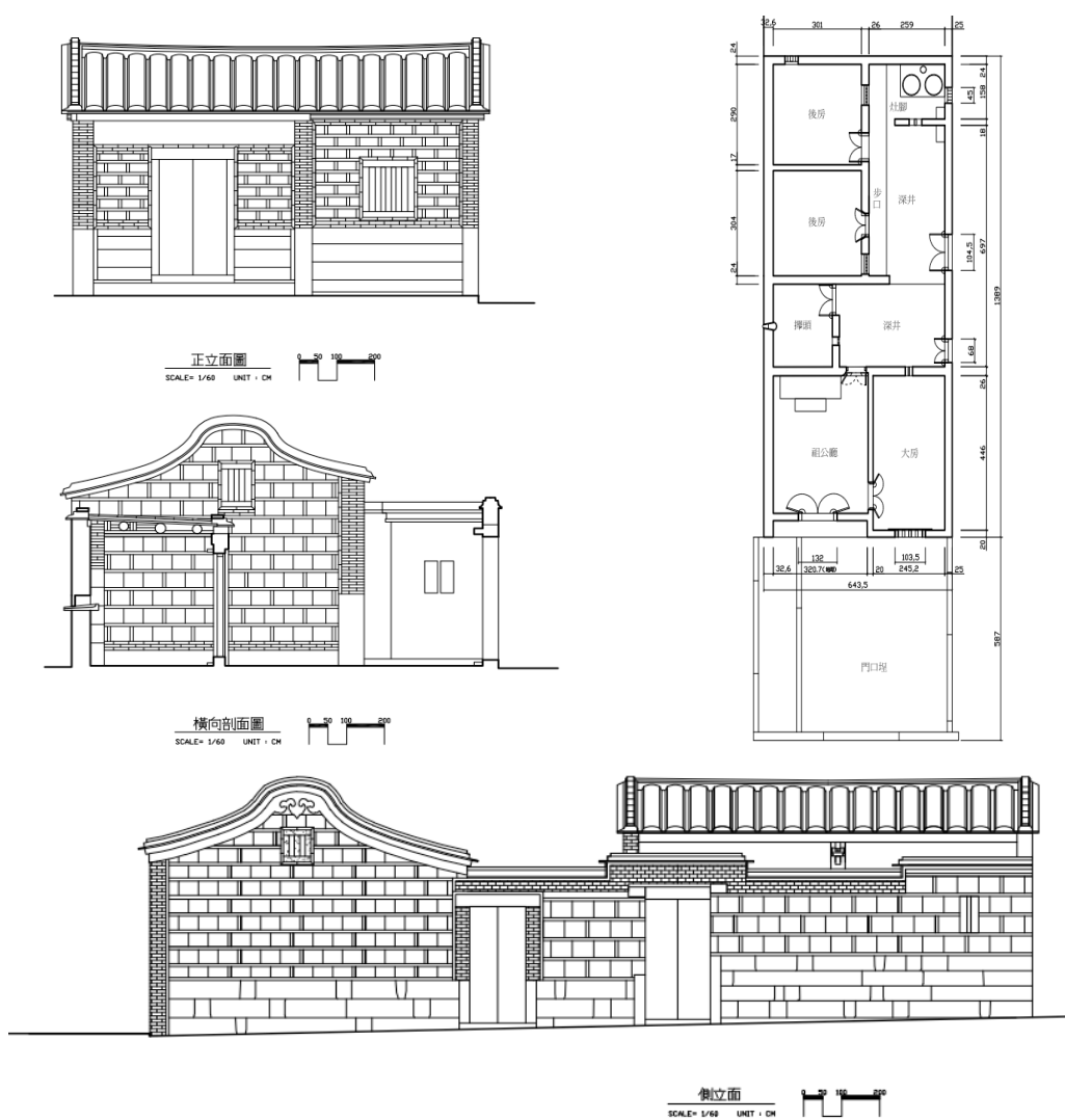
圖7 水頭黃積啟古宅基本圖
