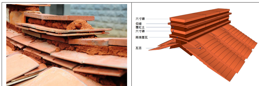
【圖68】翹筒脊
