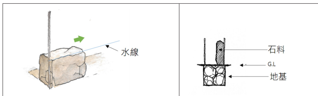
【圖28】收邊丁字砌石料依循水線砌作以確保水平
