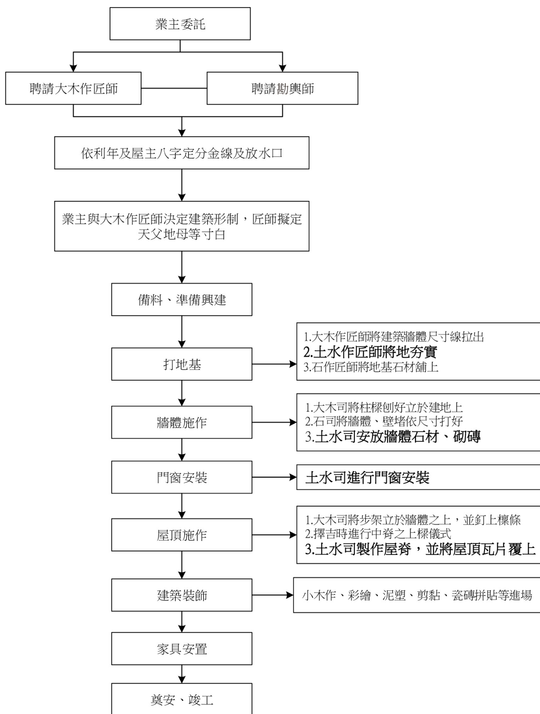
【圖1】傳統建築修繕工程施工程序圖
