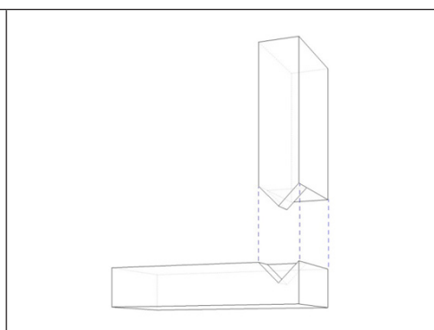
【圖56】收邊尾磚示意圖
