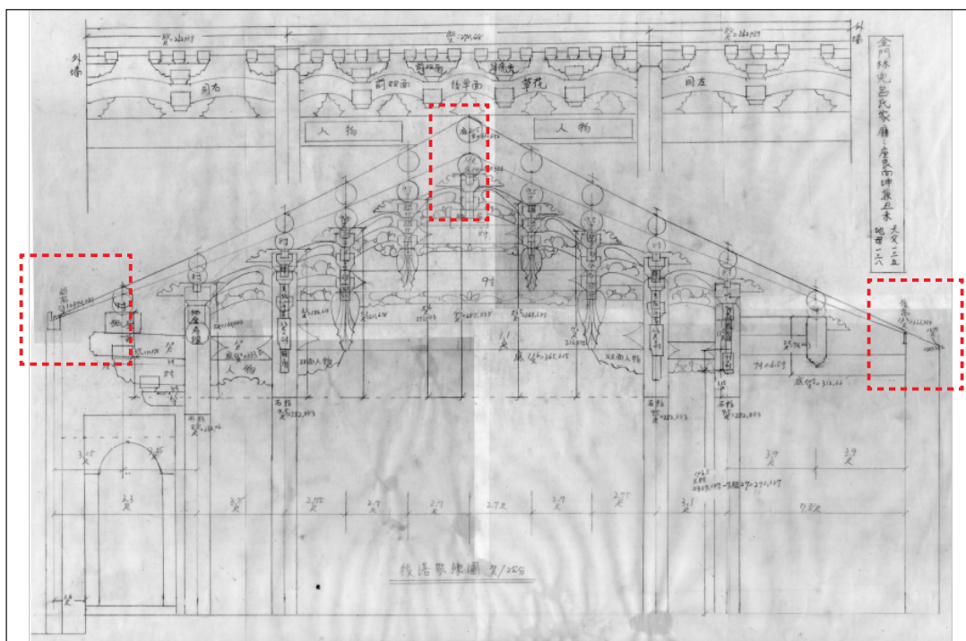
圖51 呂氏家廟後殿之天父寸白檢視
