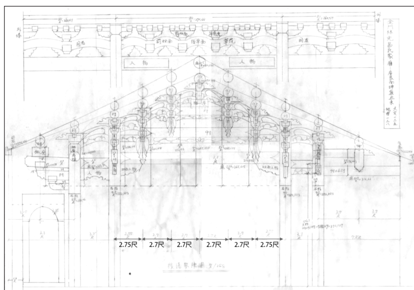
圖75 林兜林氏宗祠架內步步進（分縫尺寸）說明圖
