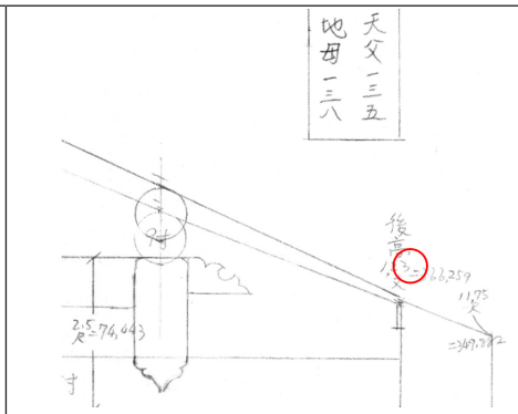
圖54 呂氏家廟後殿簷口寸白檢視
