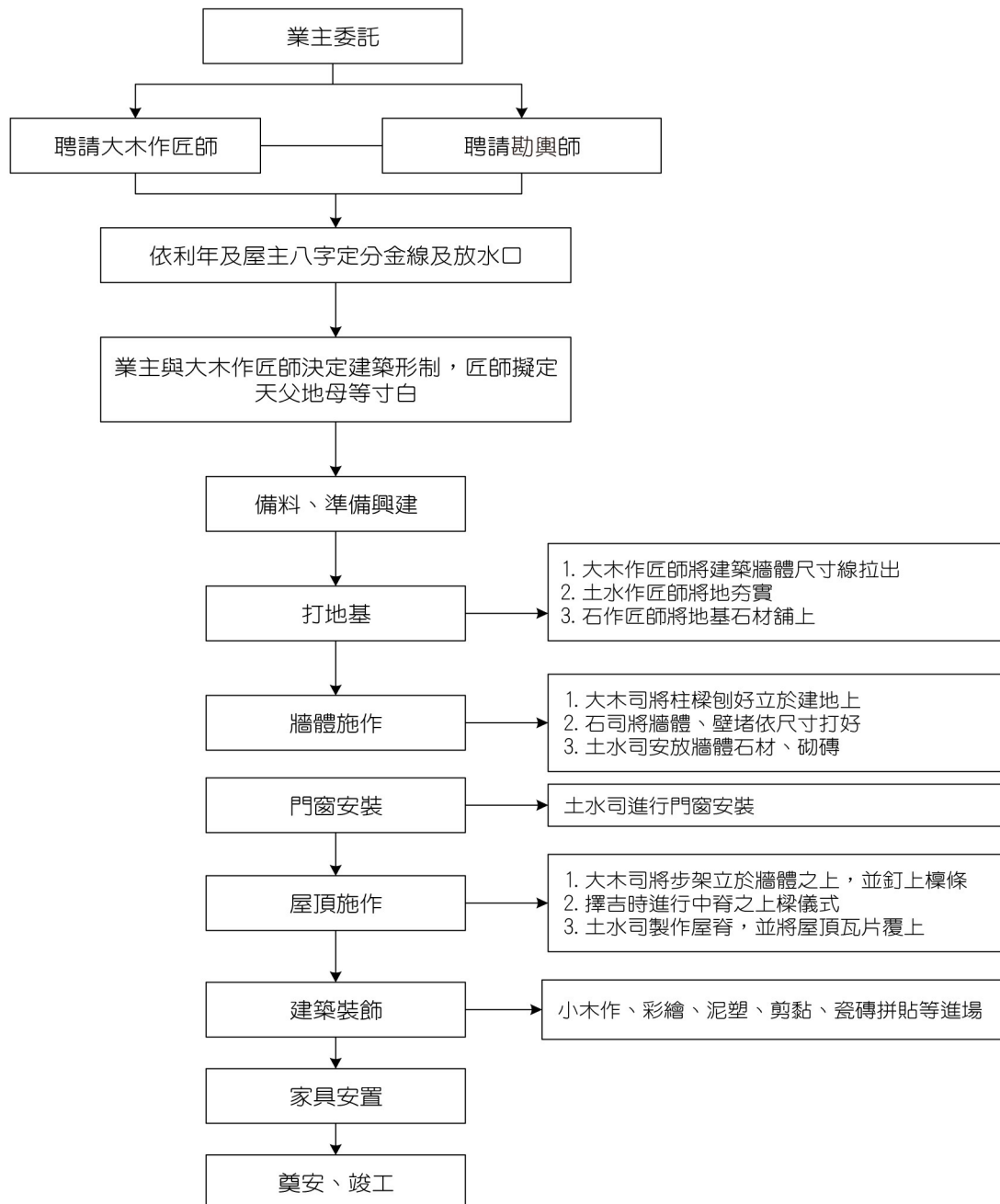
圖1 金門傳統建築營造流程圖
