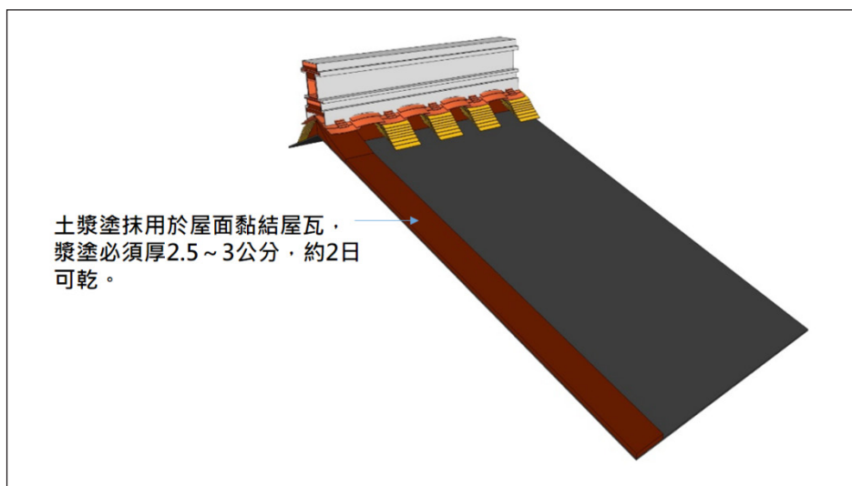
【圖13】屋面用土
