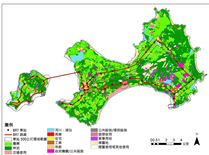
圖13 Green TOD方案B：BRT系統的建議路線和站點
