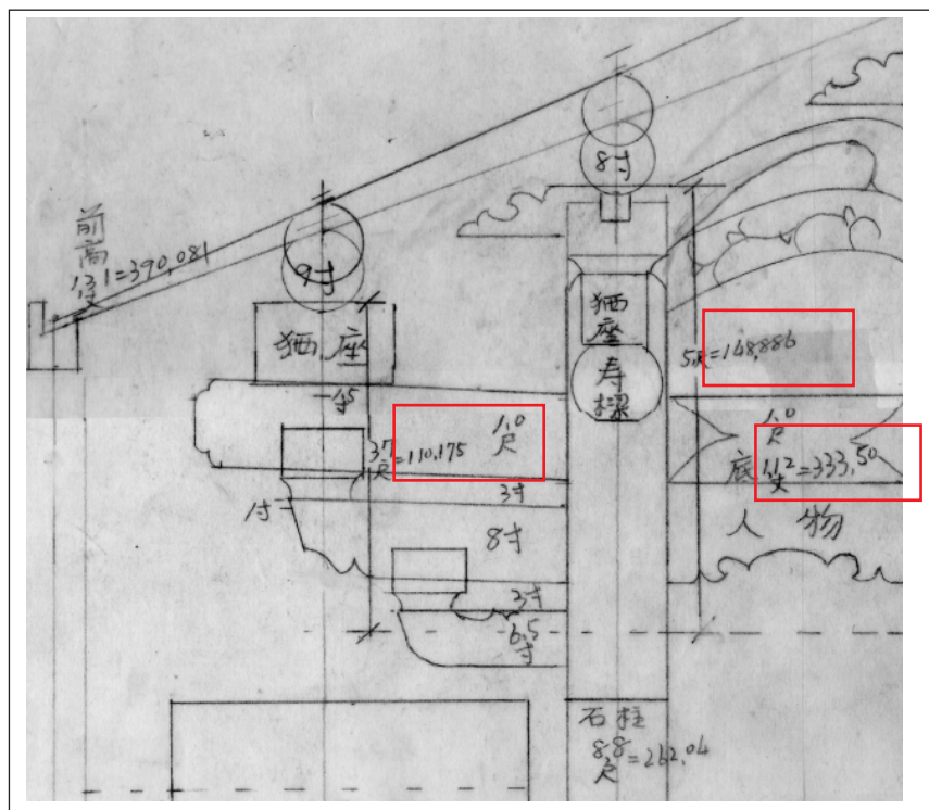
圖20 翁水千匠師繪製的棟架詳圖上的尺寸互換
