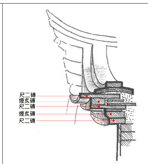
【圖64】五勻出料作法
