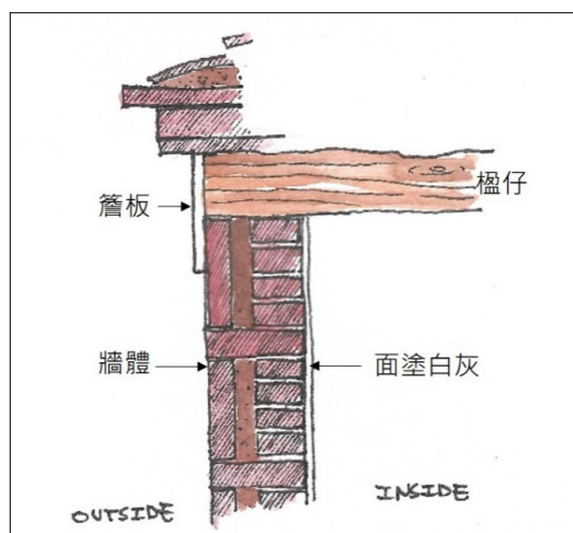
【圖59】圓規脊脊頭剖面示意
