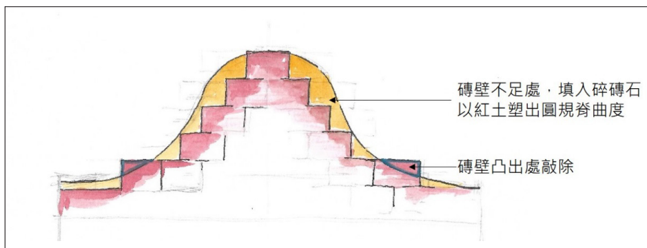
【圖57】圓規脊曲度
