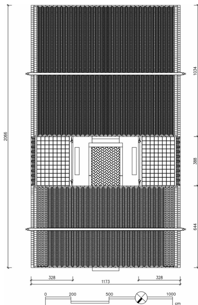
圖2-3 屋頂平面圖
